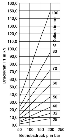
Druckkraftdiagramm für einfach- und doppelwirkende Zylinder (Wirkungsgrad 95%)
