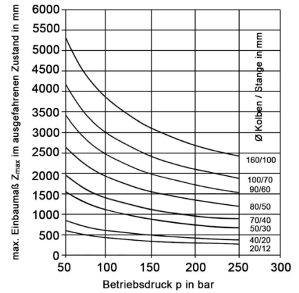
Knickungsdiagramm für einfach- und doppelwirkende Zylinder (Knicksicherheit 3,5)
