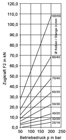
Zugkraftdiagramm für doppelwirkende Zylinder (Wirkungsgrad 92%)
