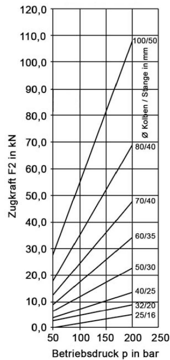
Zugkraftdiagramm für doppeltwirkende Zylinder (Wirkungsgrad 92%)
