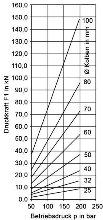
Druckkraftdiagramm für einfach- und doppeltwirkende Zylinder (Wirkungsgrad 95%)
