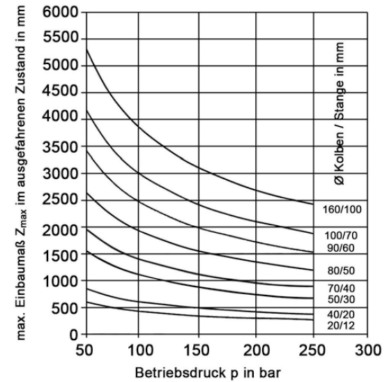
Knickungsdiagramm für einfach- und doppeltwirkende Zylinder (Knicksicherheit 3,5)
