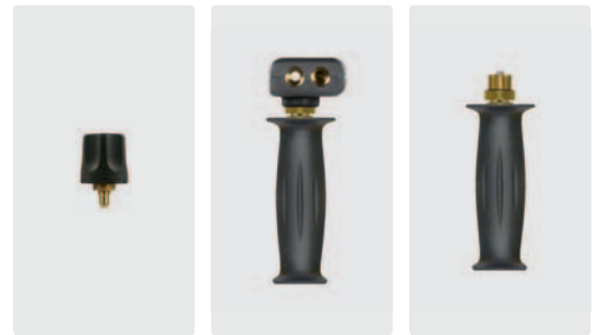
Reparatursatz ST-53 Ventil seitlich. Max. 250 bar / 150 °C Reparatursatz ST-54
