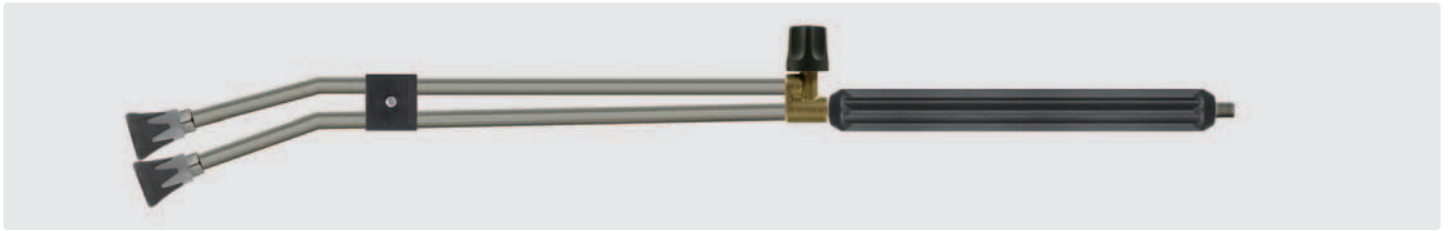
1/4" AG. Strahlrohr mit umpritzter Isolierung, Ventil ST-53 oben und Düsenschutz ST-10 mit Niederdruckdüse & Muffe 1/4" IG. Max. 250 bar / 150 °C
