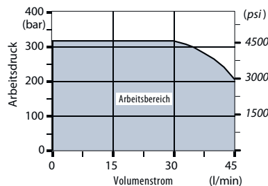
Schaltleistungsgrenze
